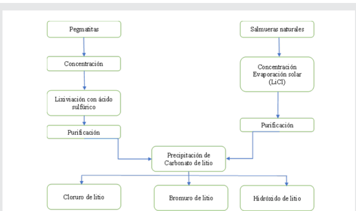
Figura 1. Procesos de extracción de litio. Fuente: Elaboración propia.
